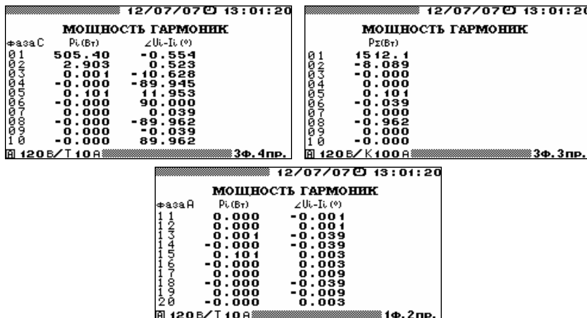
Рис. 4.12. Режим отображения гармонических составляющих активной мощности для различных схем включения
