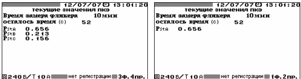
Рис. 4.23. Окна отображения кратковременной дозы фликера для трехфазной четырехпроводной и однофазной двухпроводной схем включения
