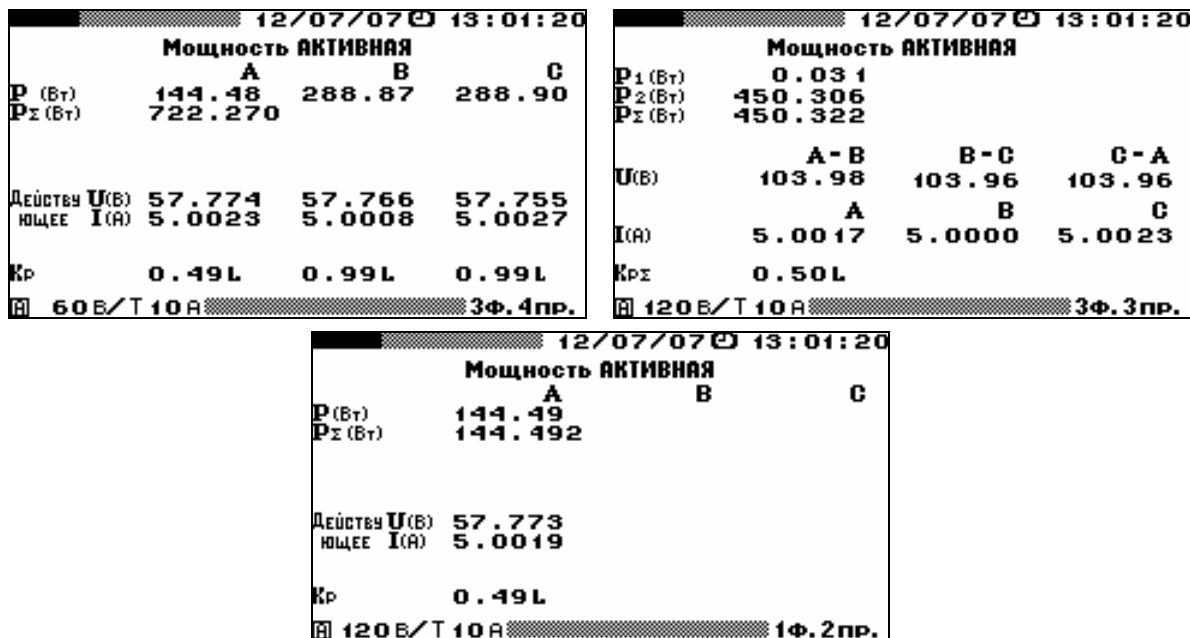
Рис. 4.6. Режим отображения активной мощности для различных схем включения
