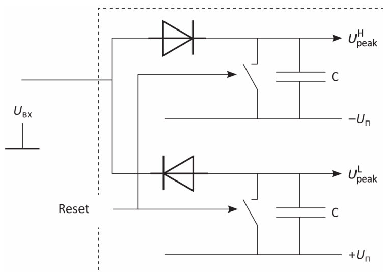
Рис. 4.50. Принцип обработки входного сигнала в режиме «ПИКОВЫЙ ДЕТЕКТОР»: U_{вх} — входное напряжение; f_s — частота дискретизации (12,8 кГц); Reset — сигнал сброса программного пикового детектора 1,25; 2,5; 5 или 10 с (выдается по программному таймеру в соответствии со значением «ВРЕМЯ УСРЕДНЕНИЯ», установленным в режиме «НАСТРОЙКИ» (см. п. 4.10.6)); U_{peak}^H — максимальное зафиксированное значение напряжения; U_{peak}^L — минимальное зафиксированное значение напряжения; C — элемент памяти программного пикового детектора; -U_{п} — минимально возможное напряжение; +U_{п} — максимально возможное напряжение
