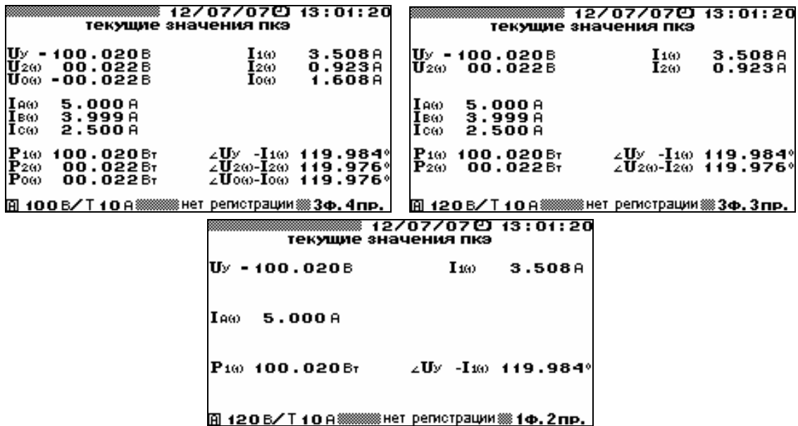
Рис. 4.22. Окна отображения токов и мощностей прямой, обратной и нулевой последовательностей для различных схем включения
