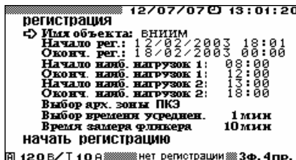
Рис. 4.16. Запрос на подтверждение начала регистрации
